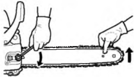
Неправильное натяжение
